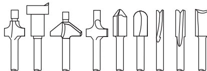
Embout (fers) de toupie en acier rapide
